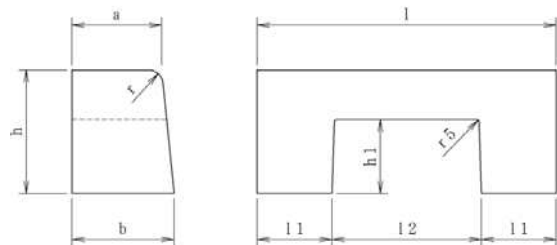
水抜きブロック 片面
