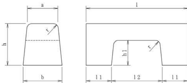
水抜きブロック 両面
