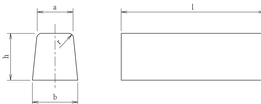
両面歩車道境界ブロック
