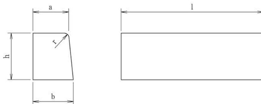
片面歩車道境界ブロック
