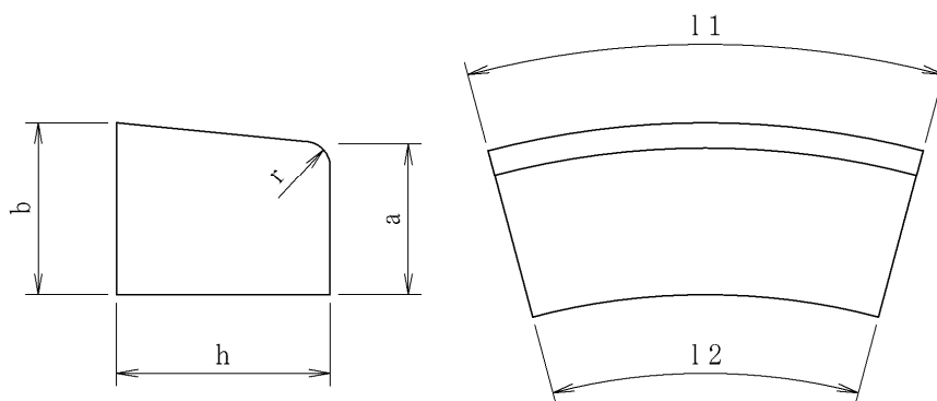
曲線部ブロック 片面B
