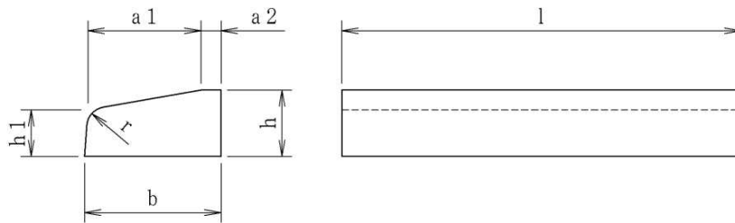
曲線部ブロック E
