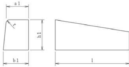
切り下げ部（乗入）ブロック 片面
