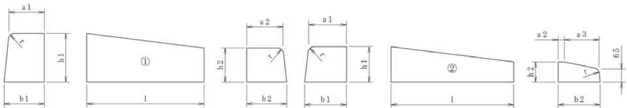
切り下げ部（乗入）2段落しブロック 片面
