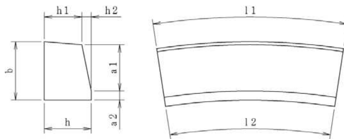
曲線部ブロック E
